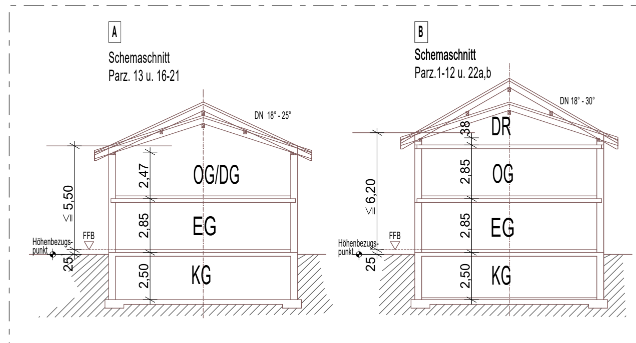
SCHEMASCHNITTE M 1:200
